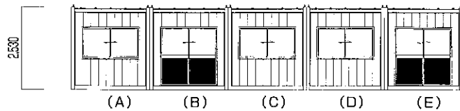
正面図
