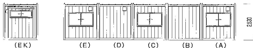
背面図
