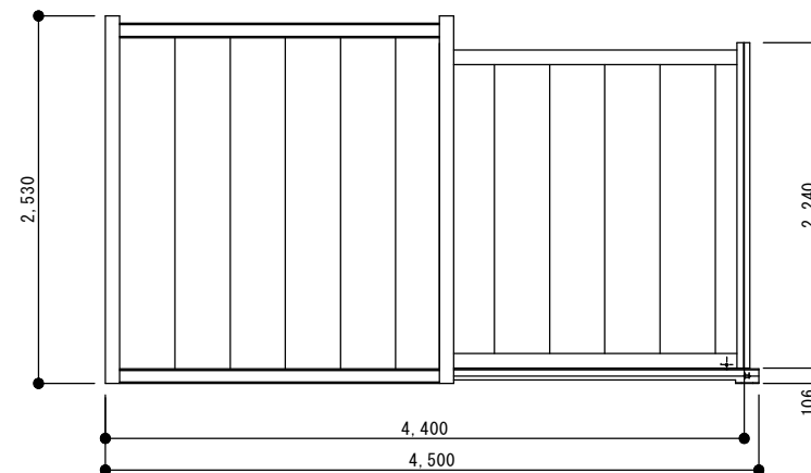
2通り立面図 S=1/20
