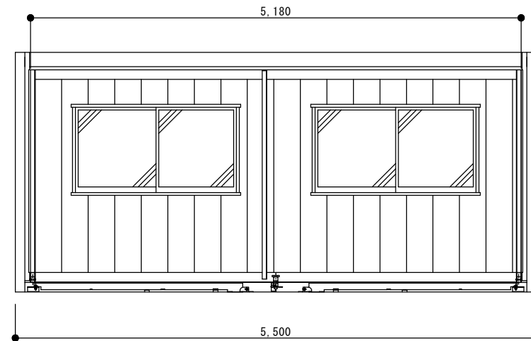
B通り立面図 S=1/20
