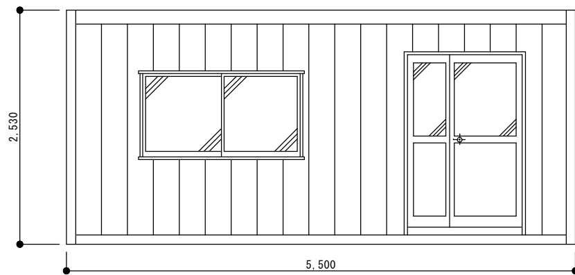
A通り立面図 S=1/20
