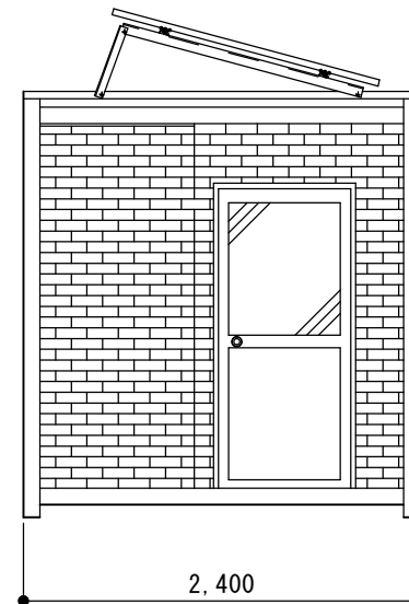
1通り 立面図 S=1/30
