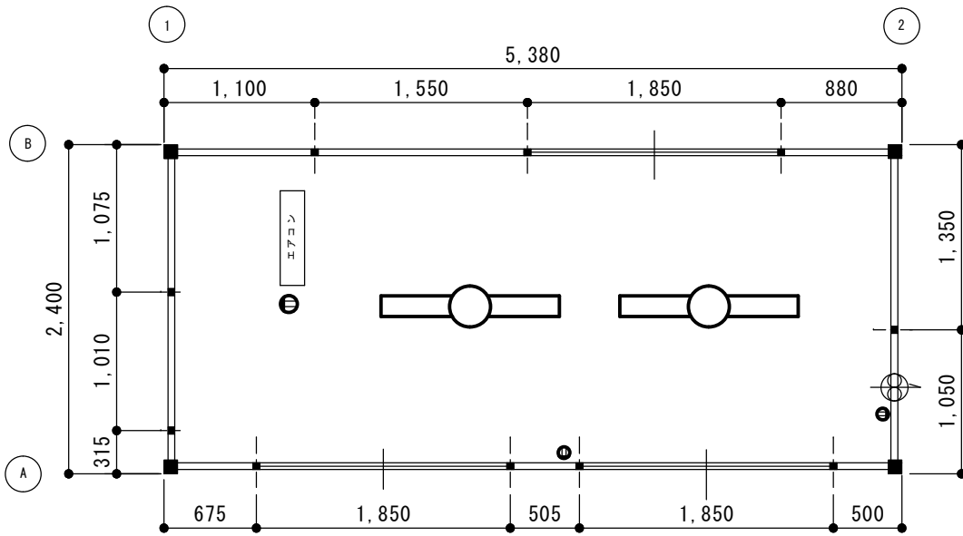
平面図 S=1/30
