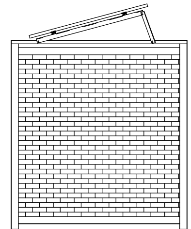
2通り 立面図 S=1/30
