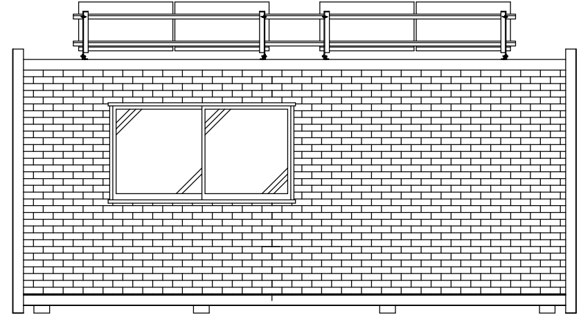
B通り 立面図 S=1/30
