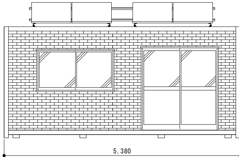
A通り 立面図 S=1/30
