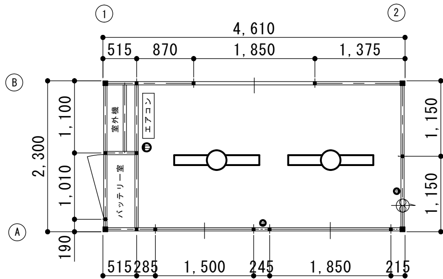
平面図 S=1/40
