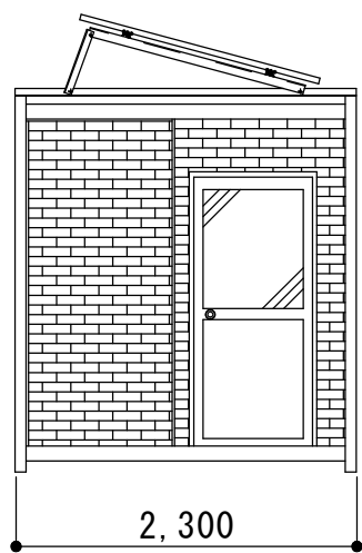
1通り 立面図 S=1/40
