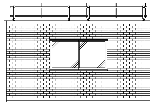
B通り 立面図 S=1/40
