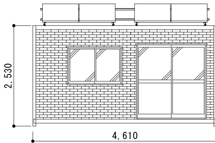
A通り 立面図 S=1/40
