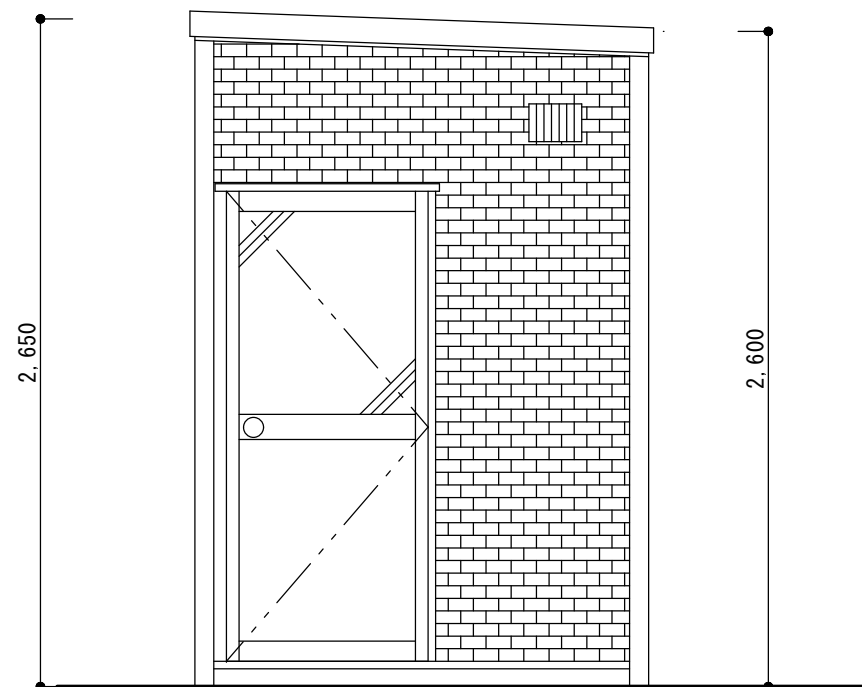
トイレハウス（洋式＋小便器＋手洗付タイプ）
